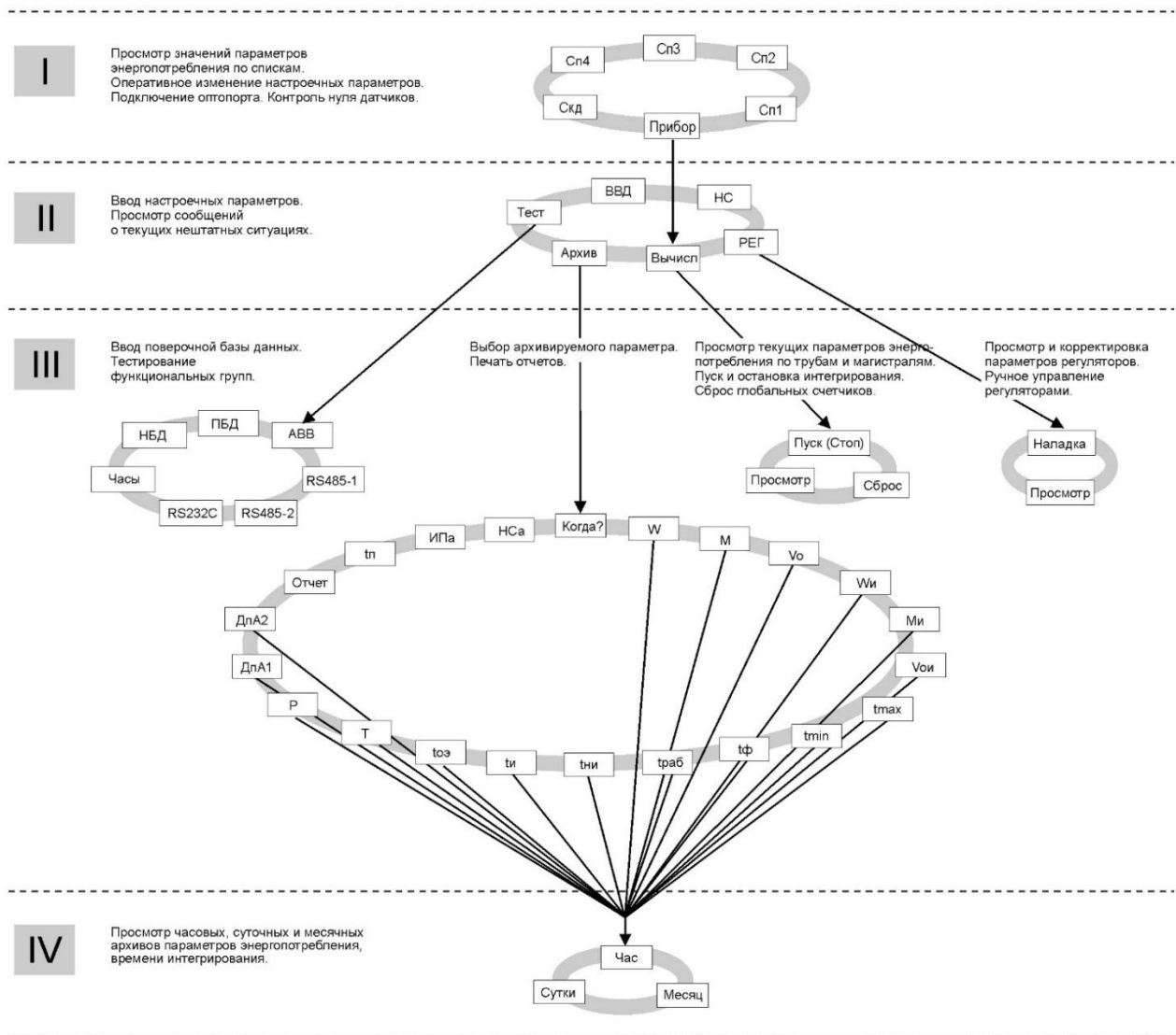
Рисунок 6.1 – Структура меню
