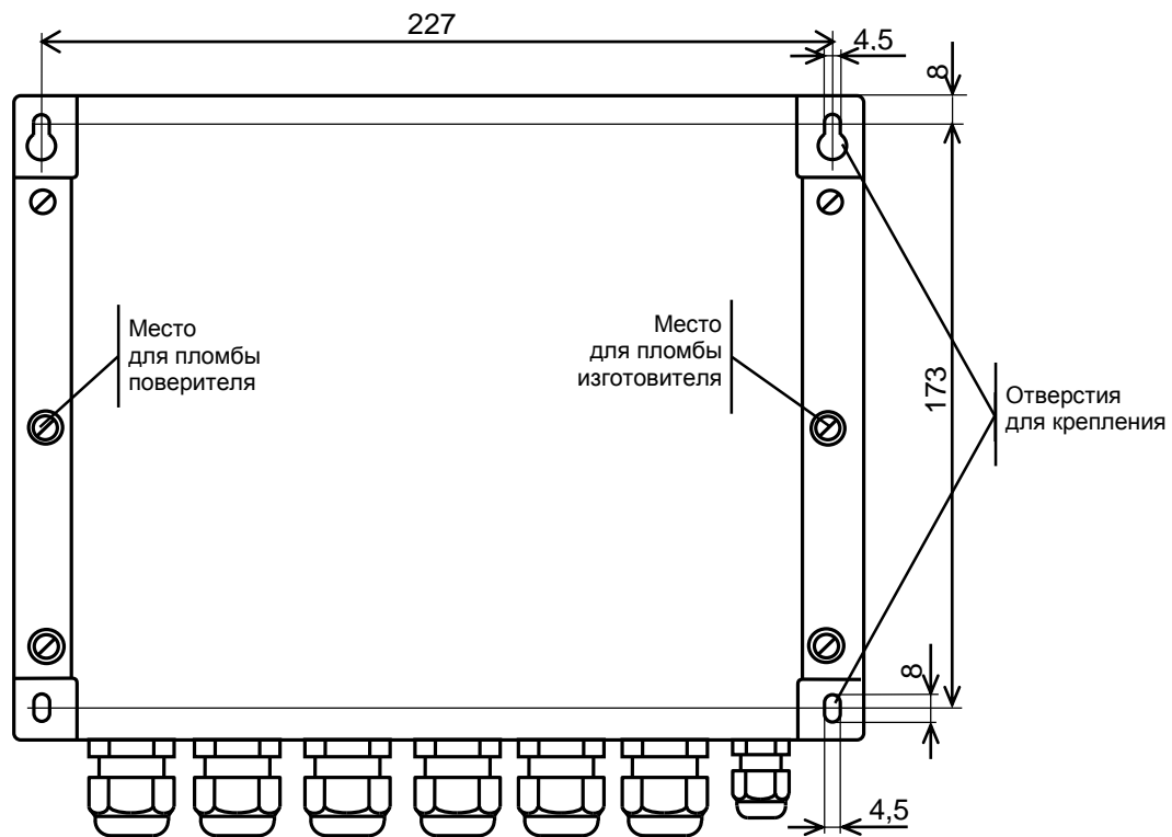
Рисунок 3.3 – Вид сзади
