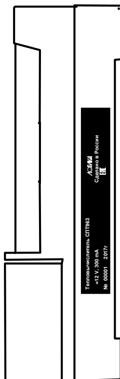
Рисунок 3.4 – Вид сбоку, кабельные вводы не показаны На боковой стороне вычислителя нанесена маркировка: тип тепловычислителя, параметры электропитания, заводской номер и год выпуска, страна – изготовитель, логотип фирмы – изготовителя, знак соответствия требованиям ЕАС
